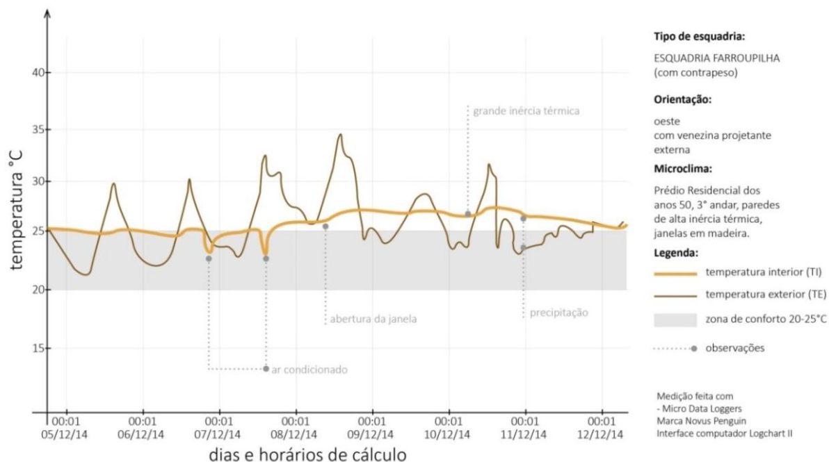
Fig. 4 - Edif. América: séries de temperatura interna e externa para a condição de verão.
