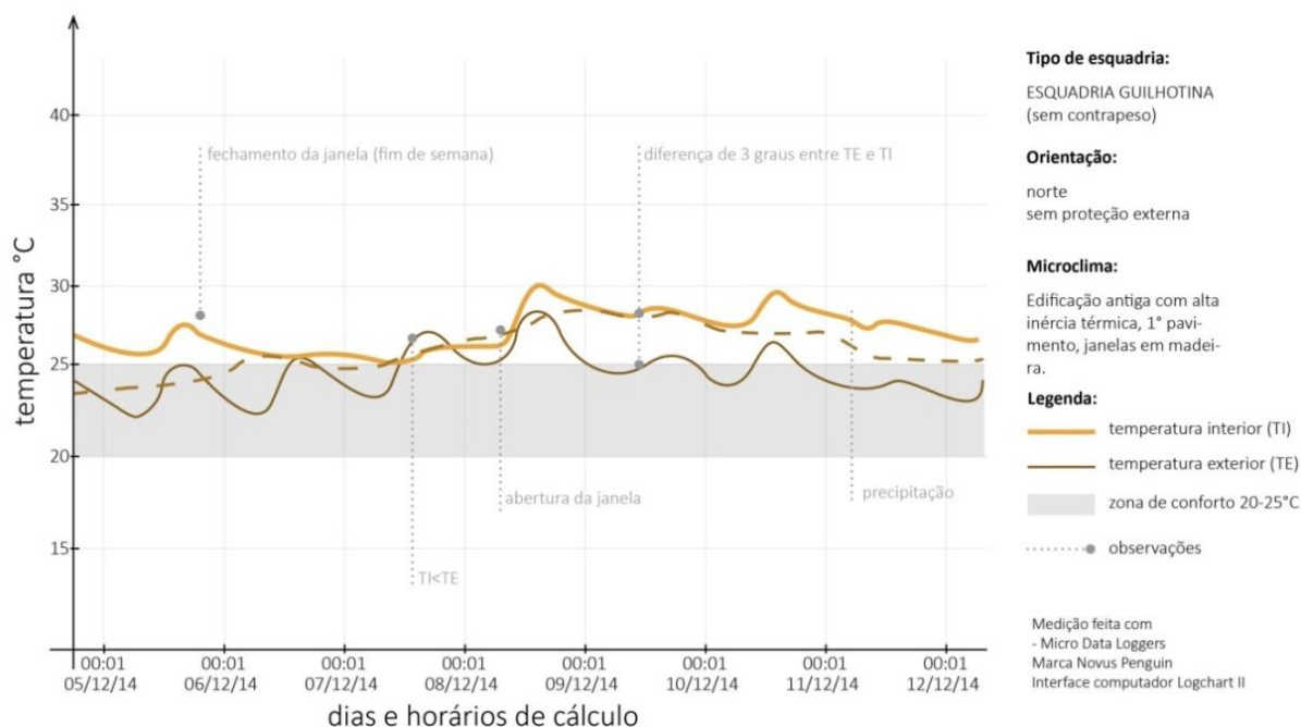
Fig. 3 - Solar da Lopo Gonçalves: séries de temperatura interna e externa para a condição de verão.
